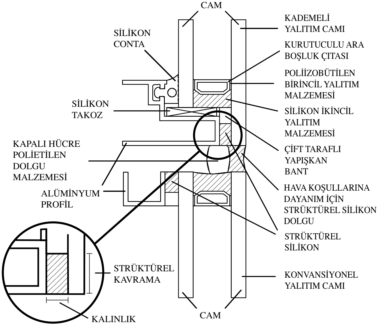
Tipik Bir Strüktürel Silikonlu Cephe Detayı
