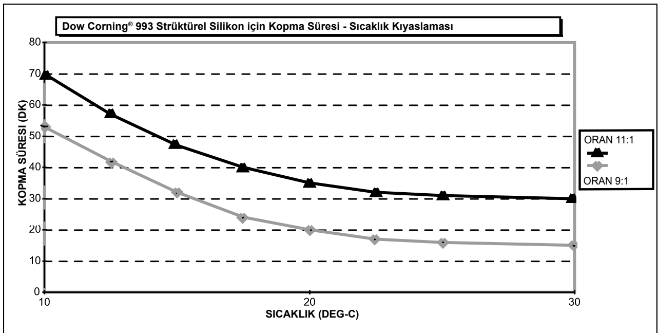
Dow Corning 993 Strüktürel Silikon için Kopma Süresi - Sıcaklık Grafiği
